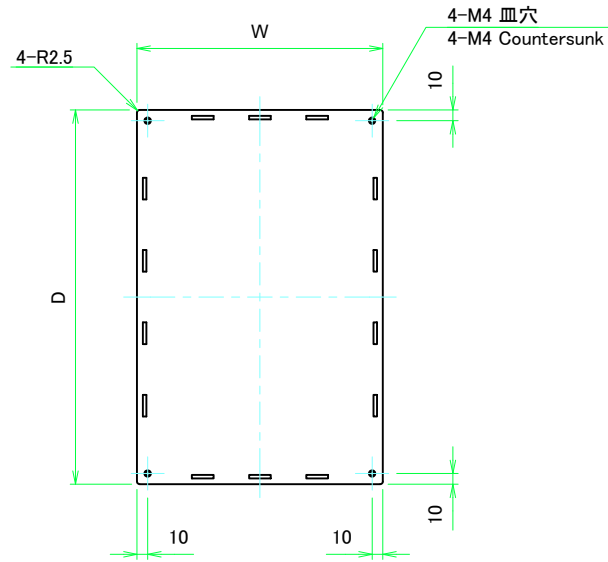
上カバー表面 / Top cover Frontside
