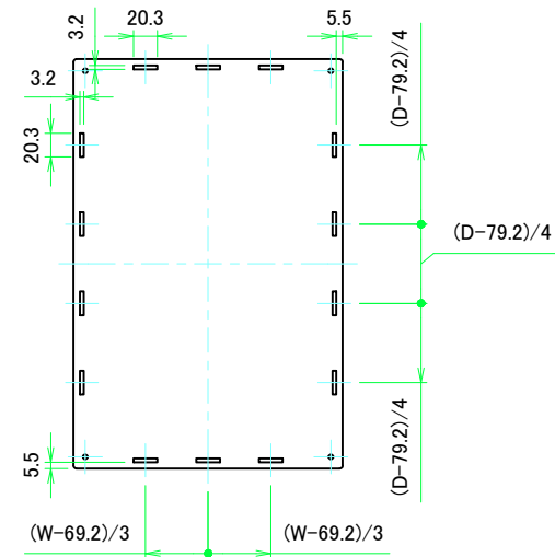
上カバー裏面 / Top cover Backside
